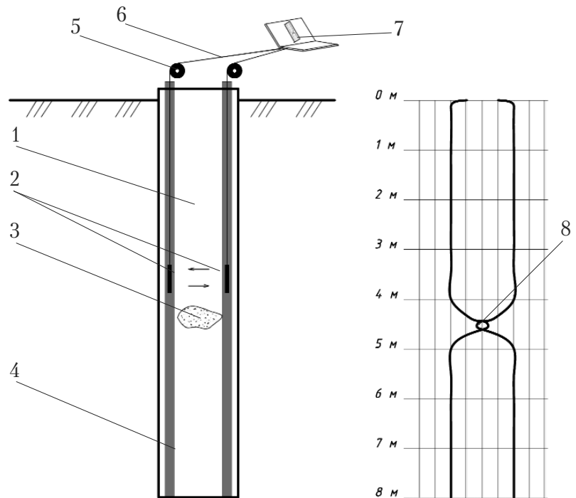
Рис. 6. Принципова схема роботи ультразвукового приладу СНУМ: 1 — досліджувана паль; 2 — ультразвукові датчики; 3 — дефект паль; 4 — заповнена водою металева труба; 5 — напрямний ролик датчика; 6 — електрокабель датчика; 7 — переносний комп'ютер; 8 — отримане на комп'ютері зображення дефекту паль
