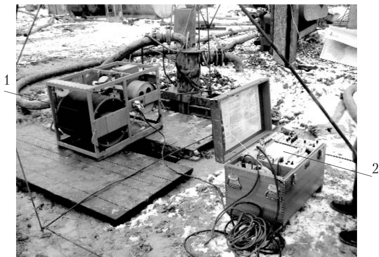
Рис. 1. Загальний вигляд бурового монітора DM-682:
